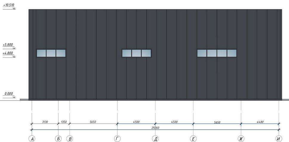
Фасад А-И
