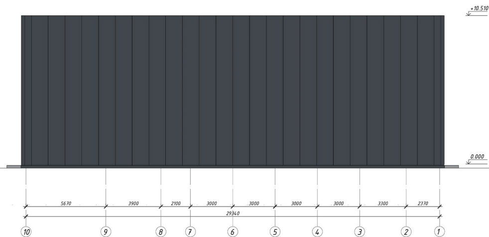
Фасад 10-1
